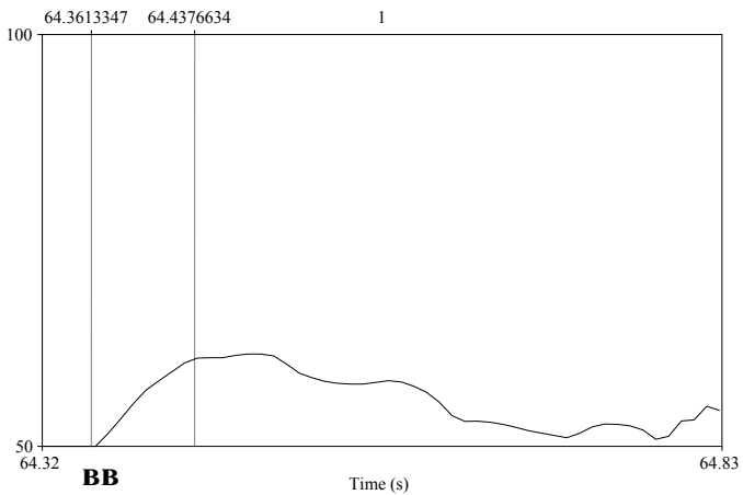
Fig. 5.7. Spectrogram of the word Ukr. 'вволене'
