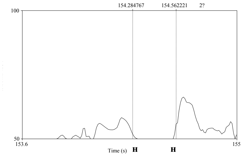
Pic. 5.3. Spectrogram of the word Ukr. 'нездола н ним'
