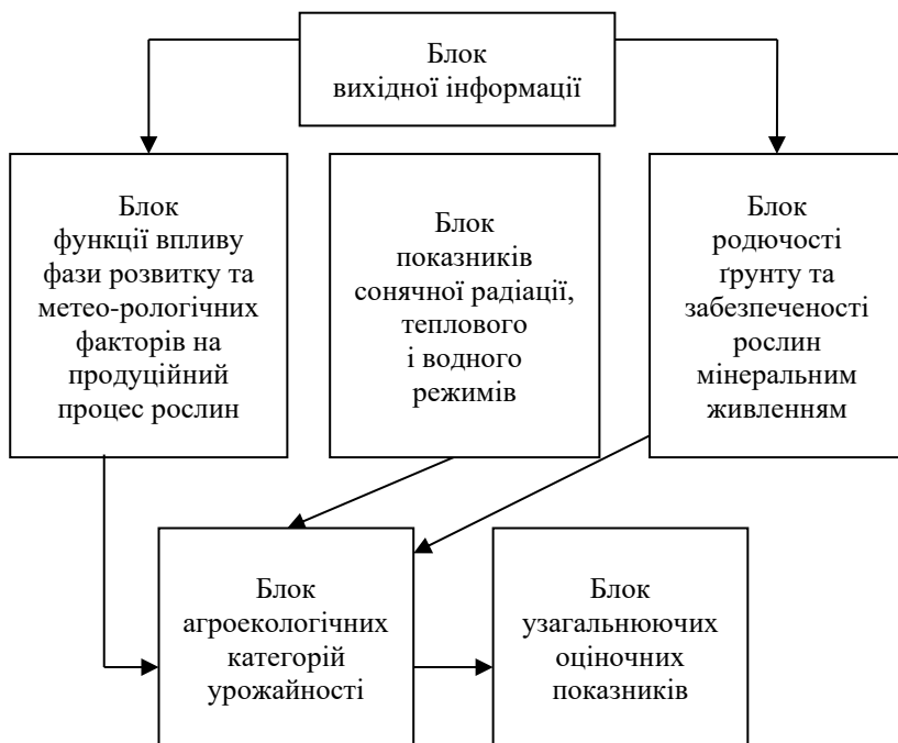
Рис. 1. Блок-схема агрокліматичної моделі формування врожаю соняшнику
