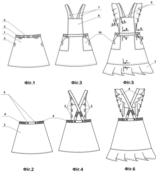
Рис. 1. Розбірний багатофункціональний предмет одягу спідниця-сарафан: фіг. 1, 2 – спідниця, фіг. 3, 4 – сарафан; фіг. 5, 6 – сарафан з крильцями та шляркою; 1-12 – деталі виробу
